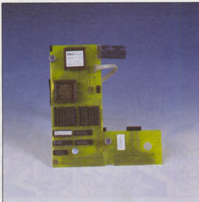
Das 2MB-Grundmodul von Richter läßt sich bis auf 14 MB erweitern
