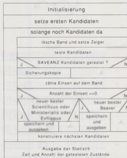
Bild 2: Die Struktur der Biberfalle
