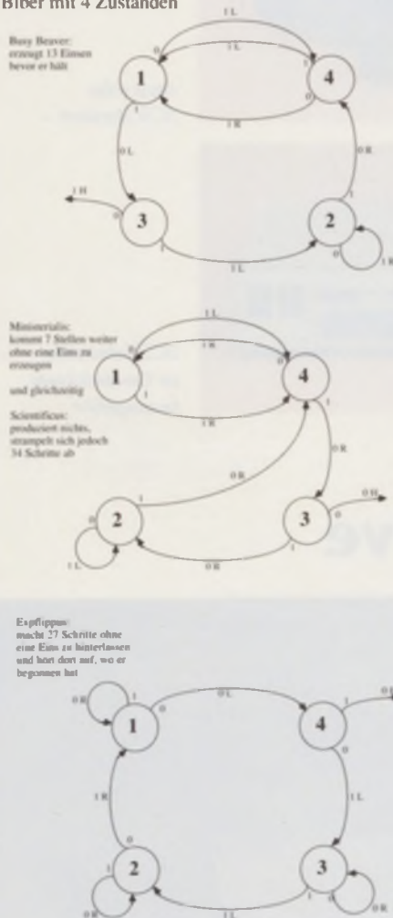
Biber mit 4 Zuständen
