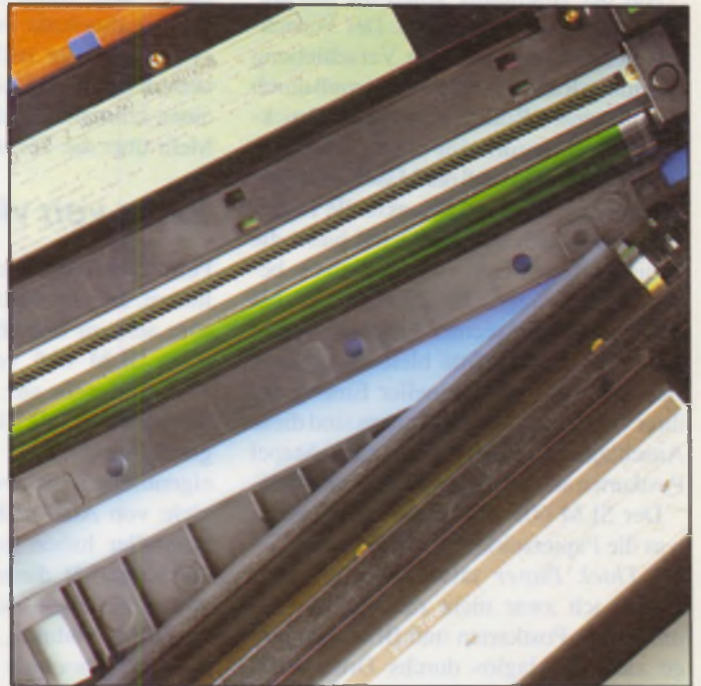
Das Herz des Lasers: Oben die grüne Bildtrommel, darunter die Entwicklereinheit. An der schwarzen Walze haftet der Toner.
