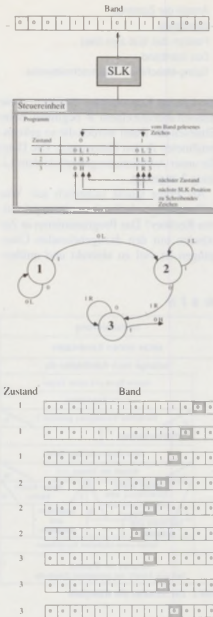
Bild 1: Die Turing-Maschine
