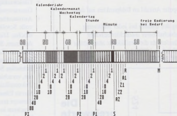
Dieses Bild zeigt die Zusammensetzung des DCF 77-Codes.
