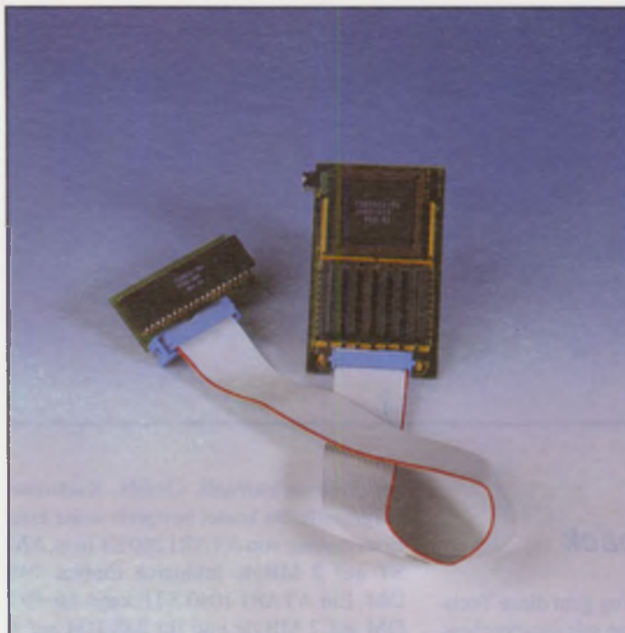
Bei der Gigatron-Erweiterung wird die MMU umgesteckt
