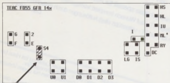
Lötbrücke offen: 80 Spuren Lötbrücke geschlossen: 40 Spuren
