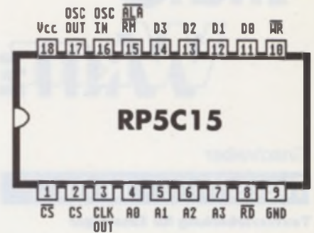
Bild 3: Die Pin-Belegung des Uhren-Chips
