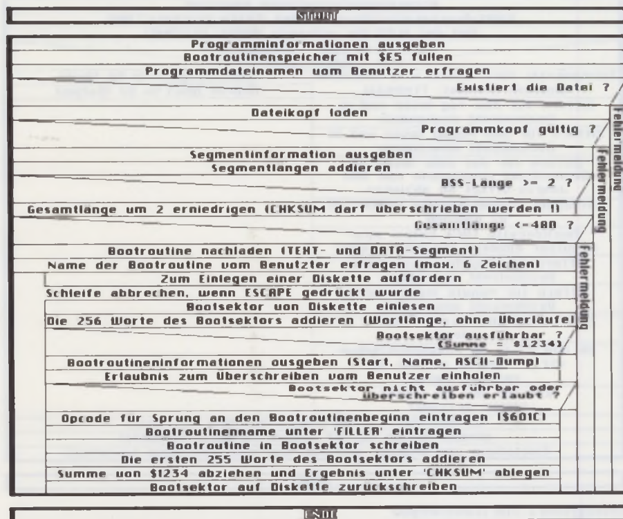
Struktogramm 1: Das Installationsprogramm
