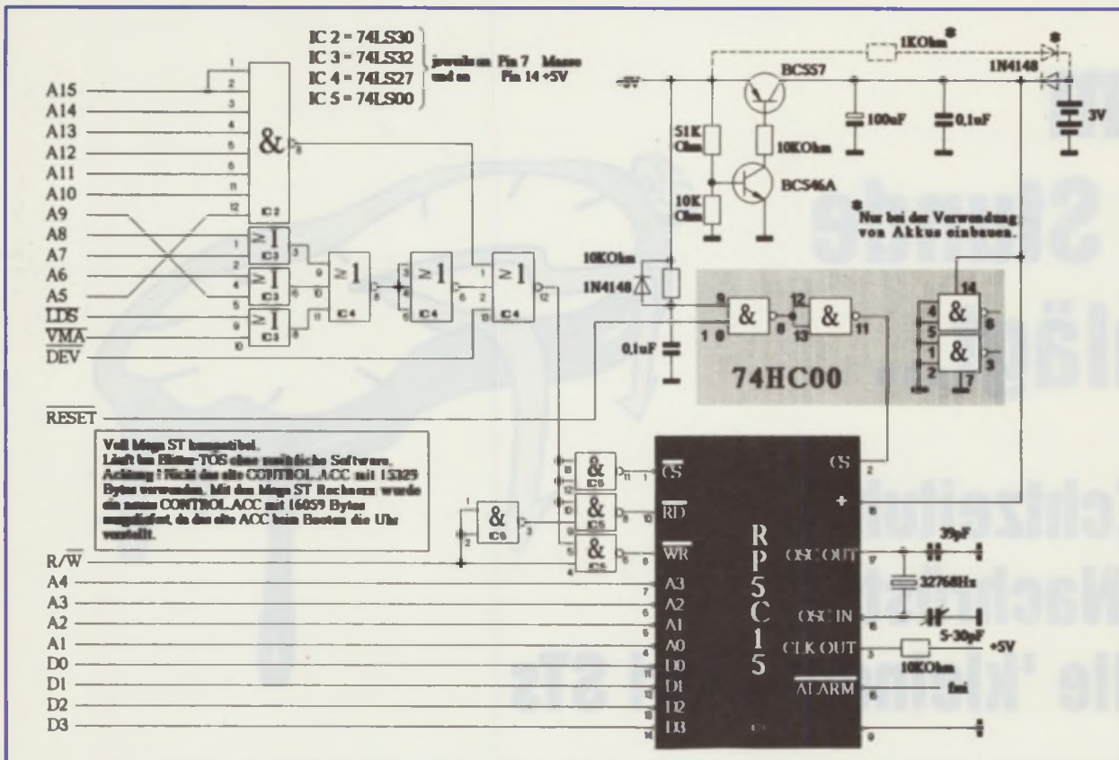
Bild 1: Der Schaltplan
