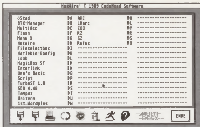
Bild 1: Das Auswahlmenü von Hotwire. Deutlich sind die Tastaturkürzel zu erkennen.
