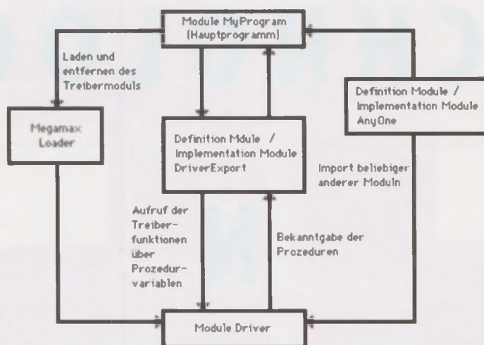
Abb.6: Funktionsbild zum Mega-Ghost-Trick.
