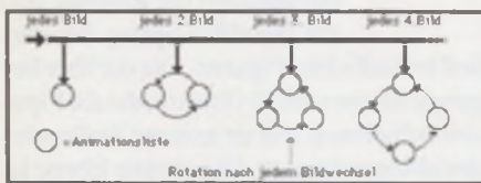
Abb.3: Verkettung der Animationslisten zur Animationsoptimierung.
