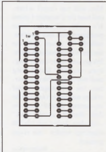
Bild 2: Platinenlayout
