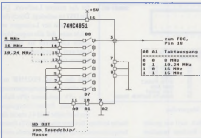
Bild 5: Pin-Belegung beim WD1772 - wichtig ist CLK!
