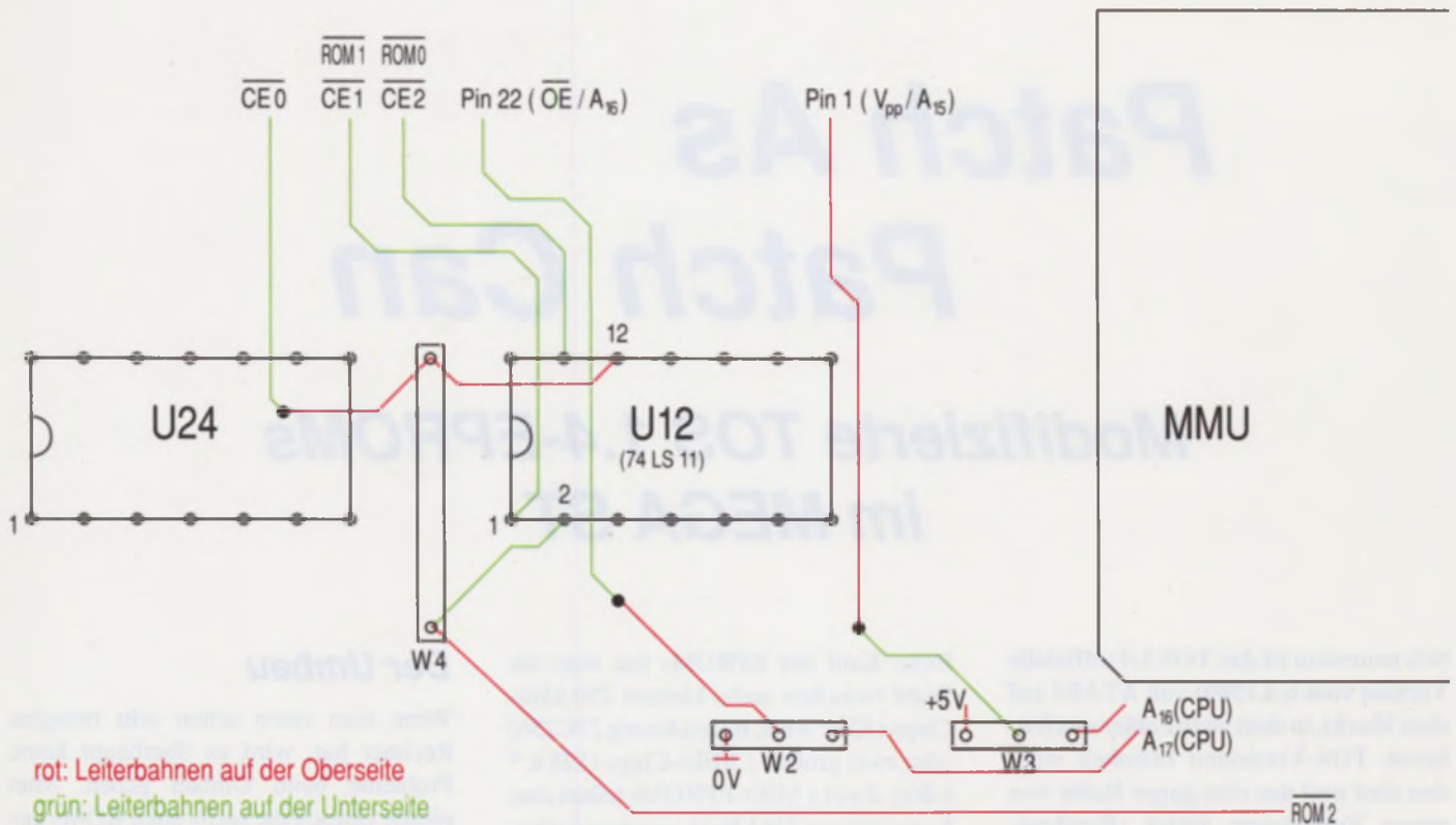
Bild 1: Änderungen am Platinenlayout, um sechs 256k- statt 2 1MB-Bit-(EP)ROMs verwenden zu können.
