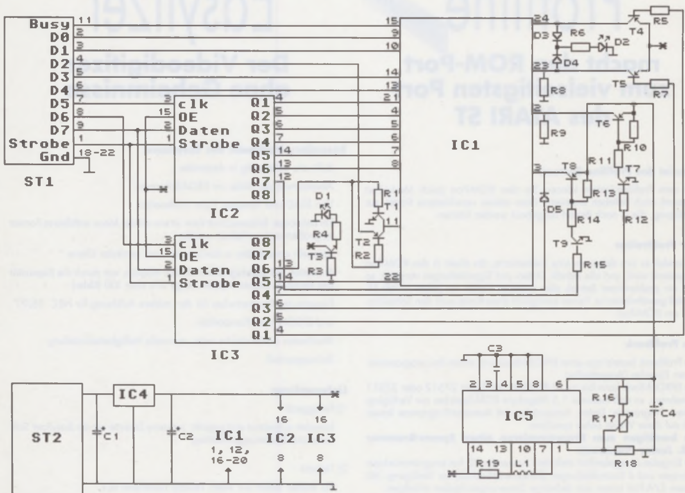
Bild 3: Schaltplan
