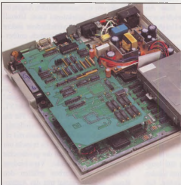
Bild 1: Eine eingebaute MGE-Grafikkarte
