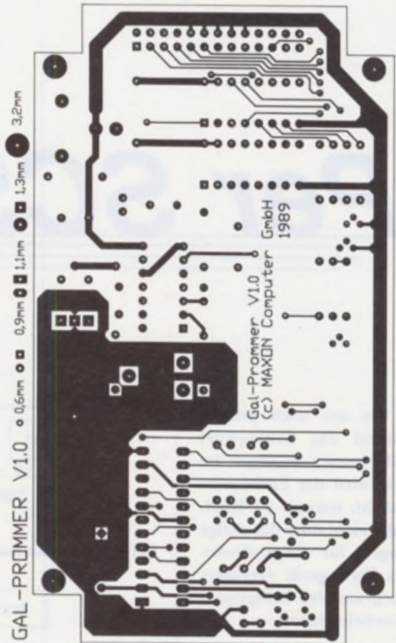
Bild 6: Bestückungsseite (1:1)
