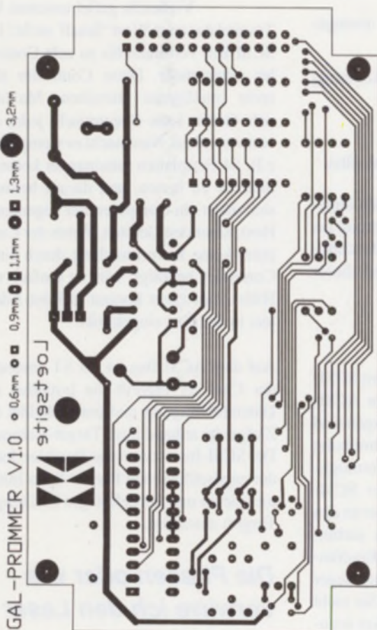
Bild 7: Lötseite (1:1)
