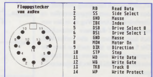
Bild 2: Floppy-Port des ST
