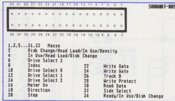
Bild 1: Pin-Belegung beim Shugart-Bus
