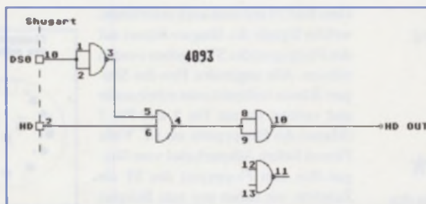
Bild 7: Das HD-Signal vom Laufwerk wird angepaßt
