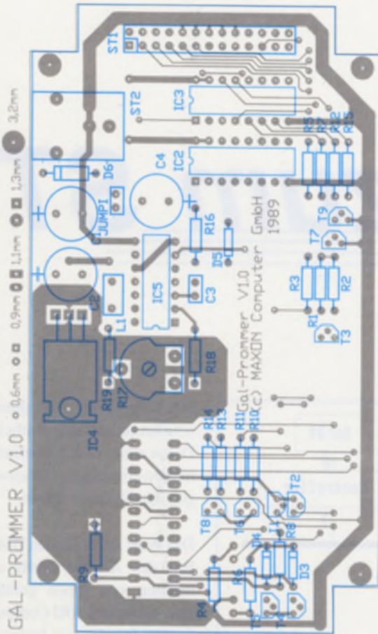
Bild 5: Bestückungsplan
