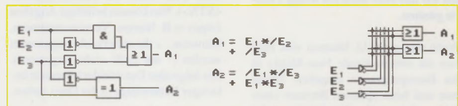
Bild 4: Verknüpfungsnetz mit TTL-Logik und im GAL
