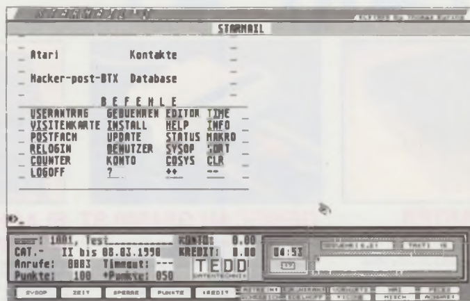
Bild 2: Starmail online
