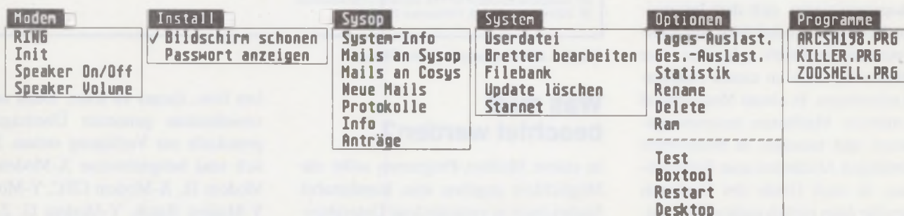
Bild 1: Die Starmail-Menüs
