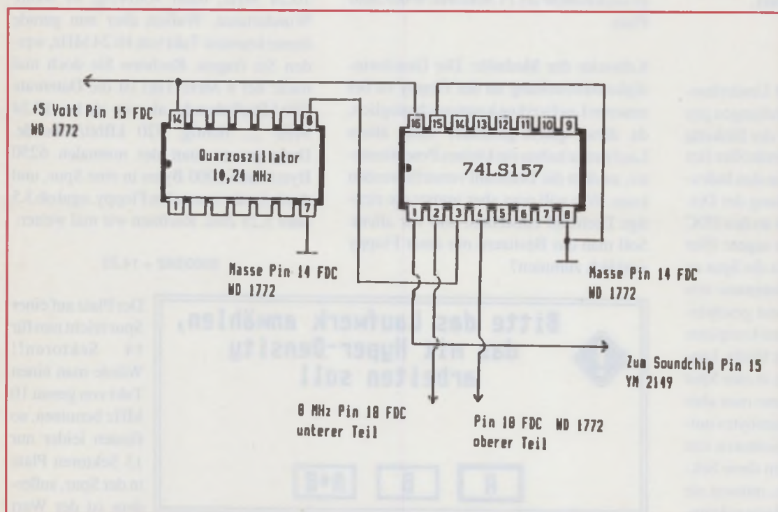
Schaltplan für Hyper-Density
