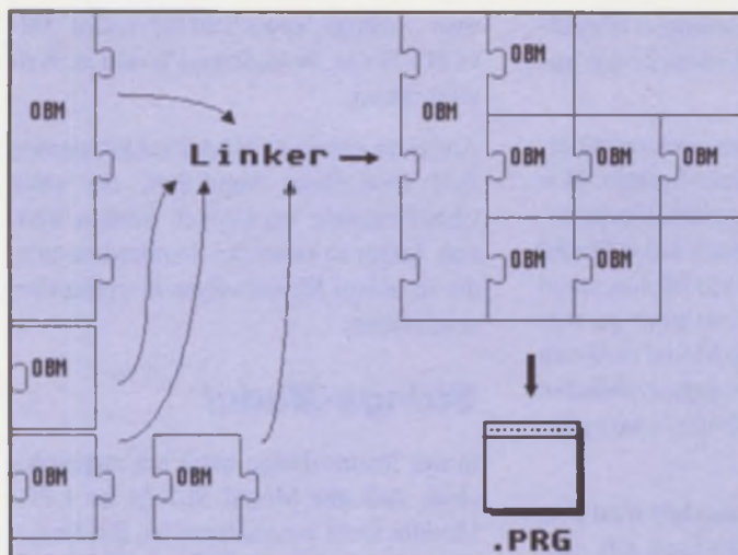
Bild 2: Zusammenbinden des Hauptprogramms mit den importierten Objektdateien.
