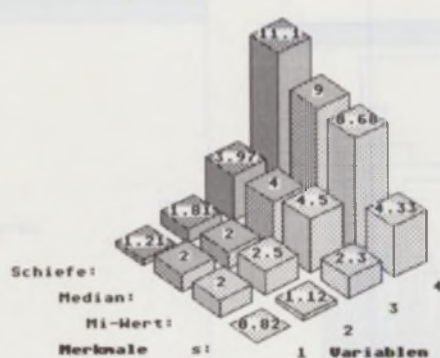
Abb. 2: ST-STATISTIK - Säulendiagramm
