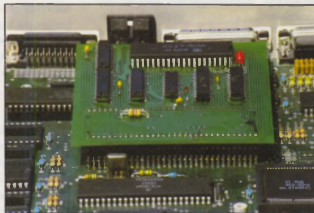
PC-Speed muß auf den Prozessor gelötet werden.
