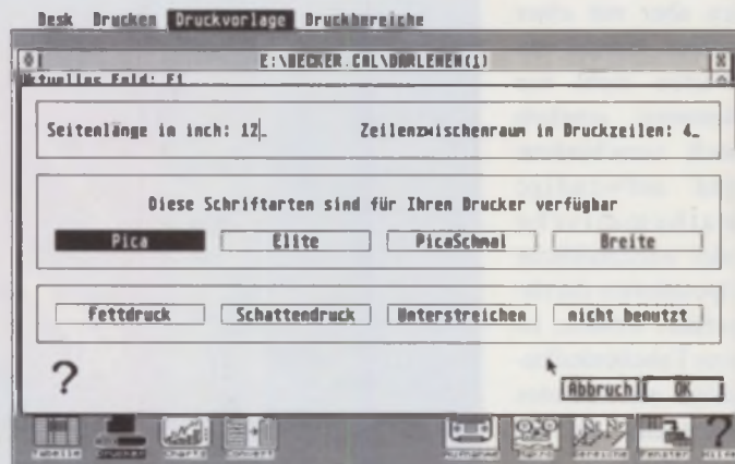
Bild 2: Die Druckdialogbox
