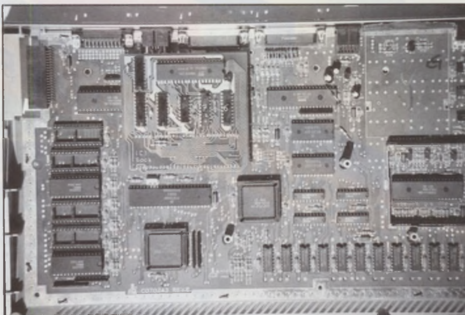
PC-Speed, der neue MS-DOS-Emulator in einem 520 ST
