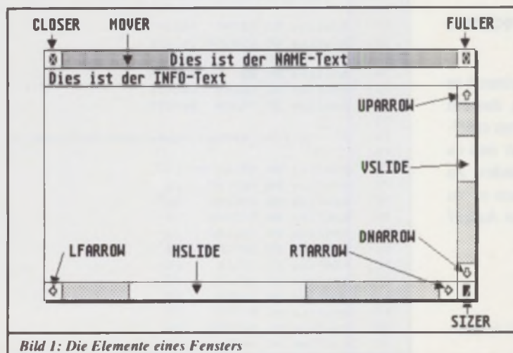
Bild 1: Die Elemente eines Fensters
