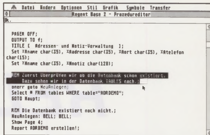
Bild 4: Erstellung der Prozedur zur Bildschirmmaske
