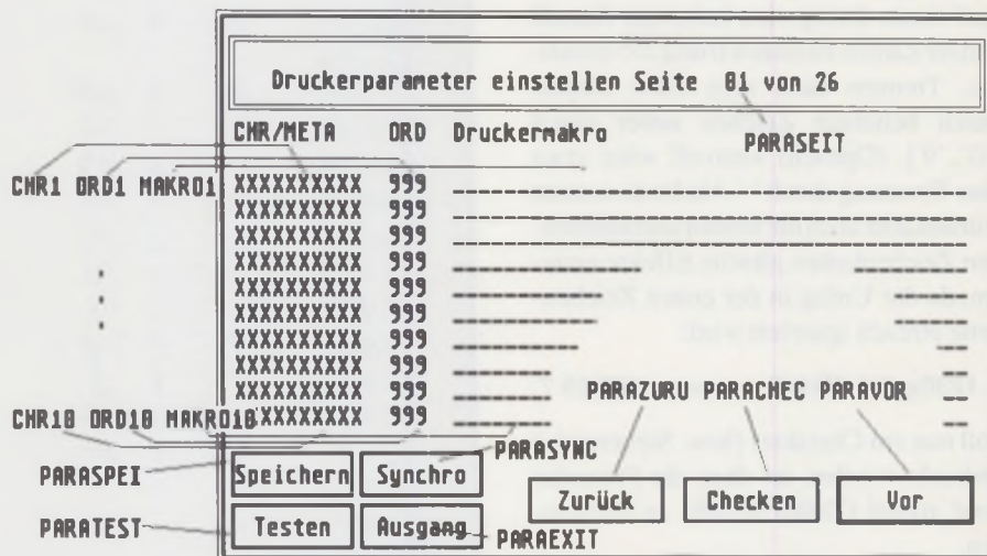
Abb. 5: Dialog "PARAMETE"
