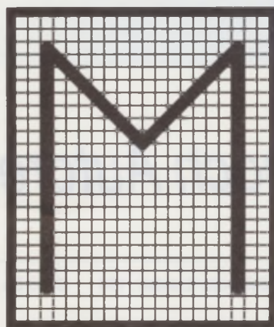
Bild 3: Das Drahtmodell-Prinzip
