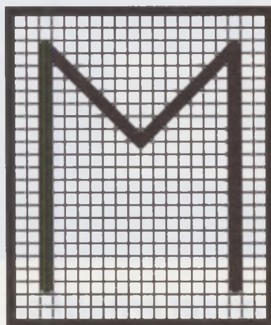
Bild 1: Das Vergleichsprinzip
