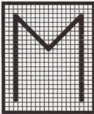
Bild 5: Das Maskenvergleichsverfahren
