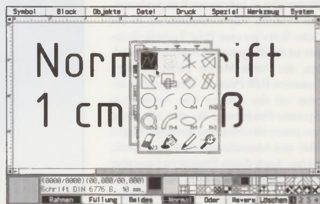
Das Pop-Up-Menü
