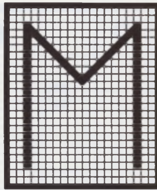
Bild 4: Das Eingrenzungsprinzip
