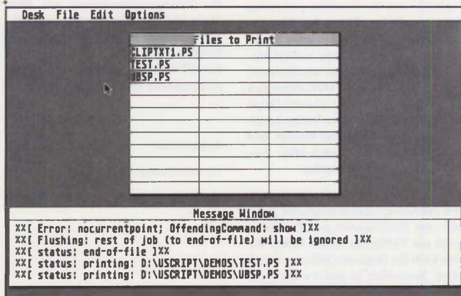
Der UltraScript-Desktop
