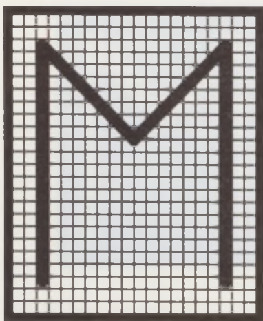
Bild 2: Das Markante-Punkte-Prinzip
