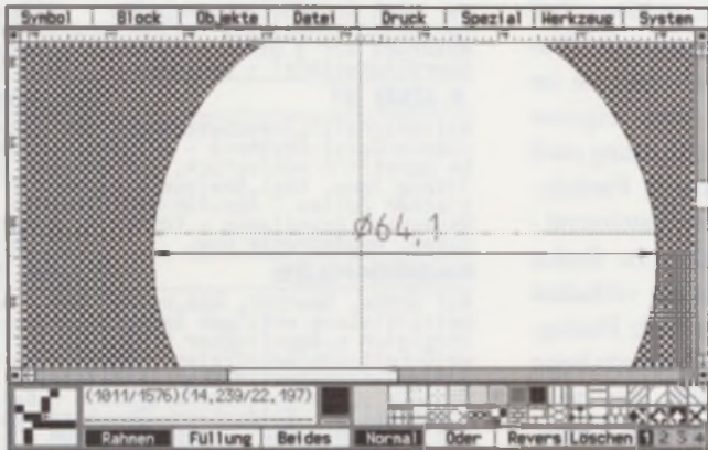
Die Bemaßungsfunktion
