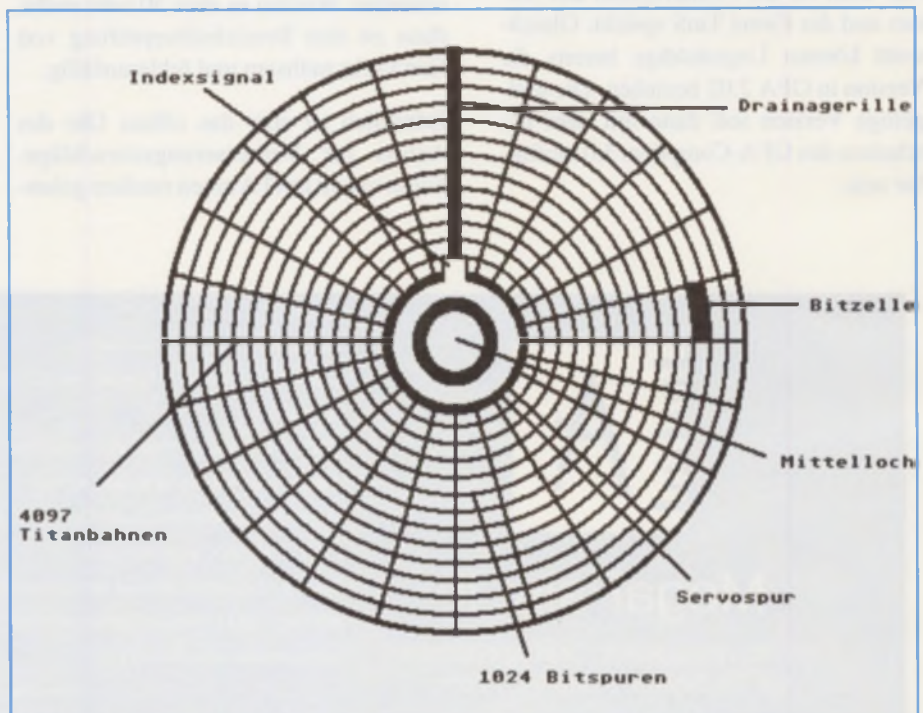
Aufbau der neuen 4 Zoll-Disketten
