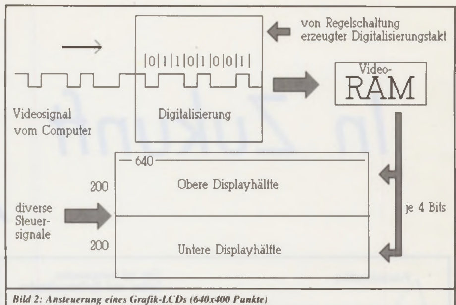
Bild 2: Ansteuerung eines Grafik-LCDs (640x400 Punkte)
