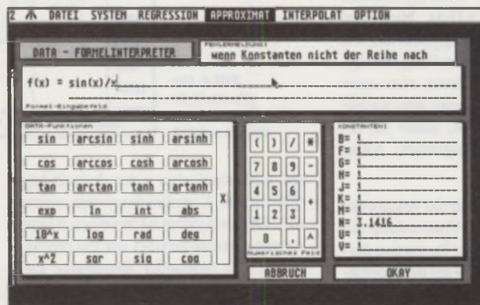
Bild 2: Eingebauter Formelinterpreter
