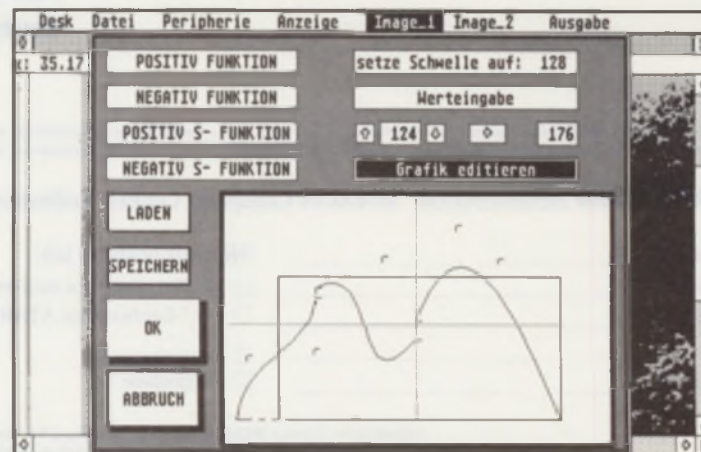
Die Transferfunktion
