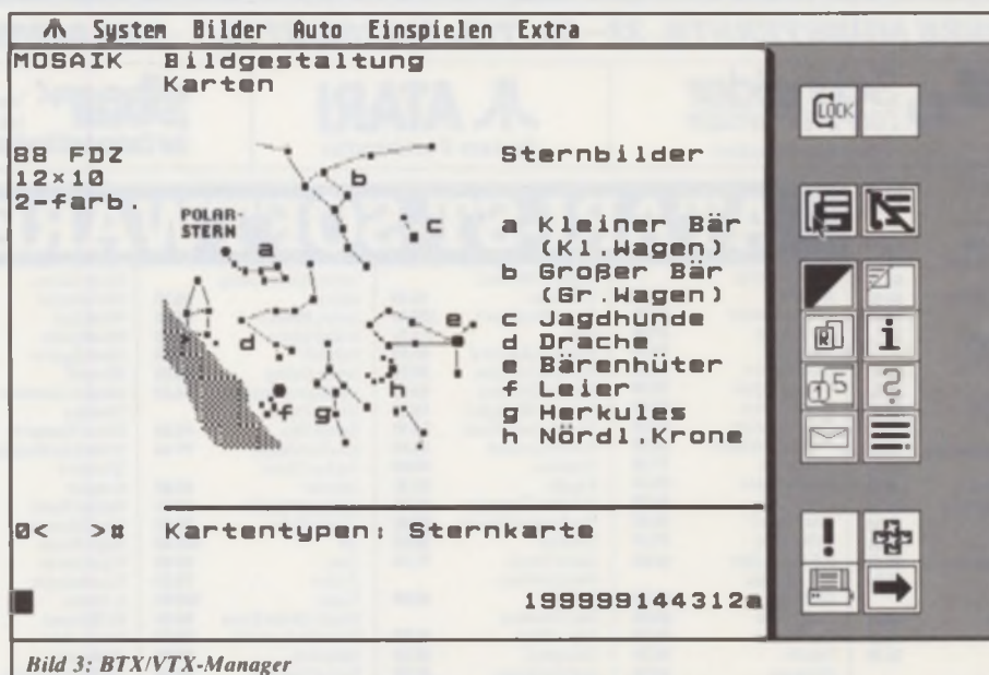
Bild 3: BTX/VTX-Manager
