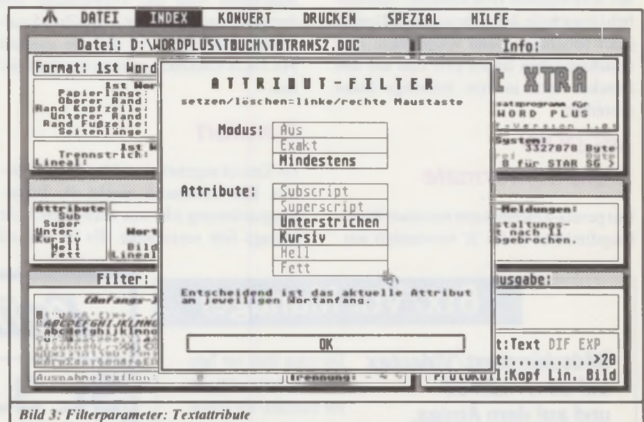
Bild 3: Filterparameter: Textattribute
