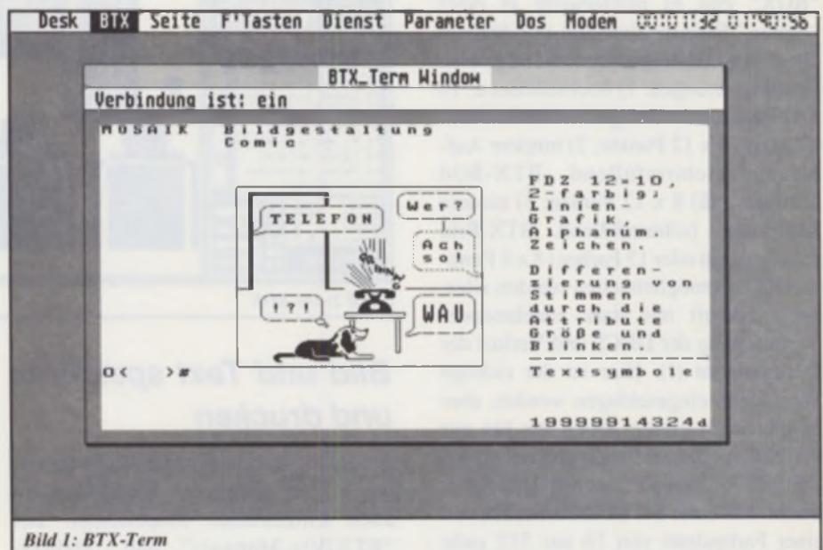
Bild 1: BTX-Term
