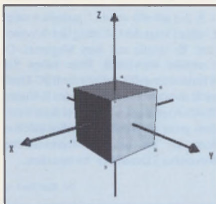
Abb.1: Würfel im kartesischen Koordinatensystem.
