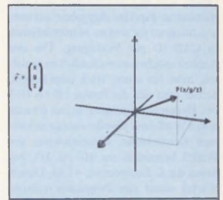
Abb. 2: Der Ortsvektor \vec{r} zum Punkt P
