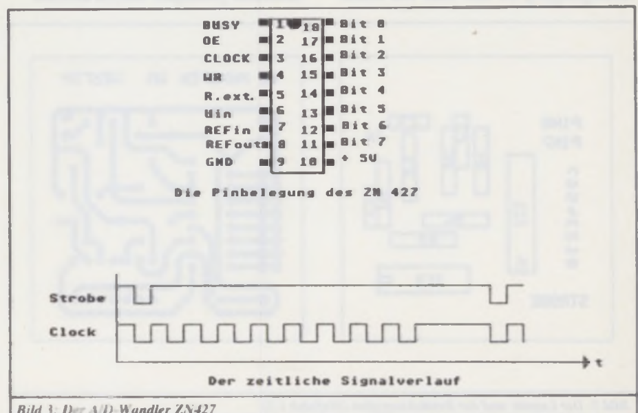
Bild 3: Der A/D-Wandler ZN427
