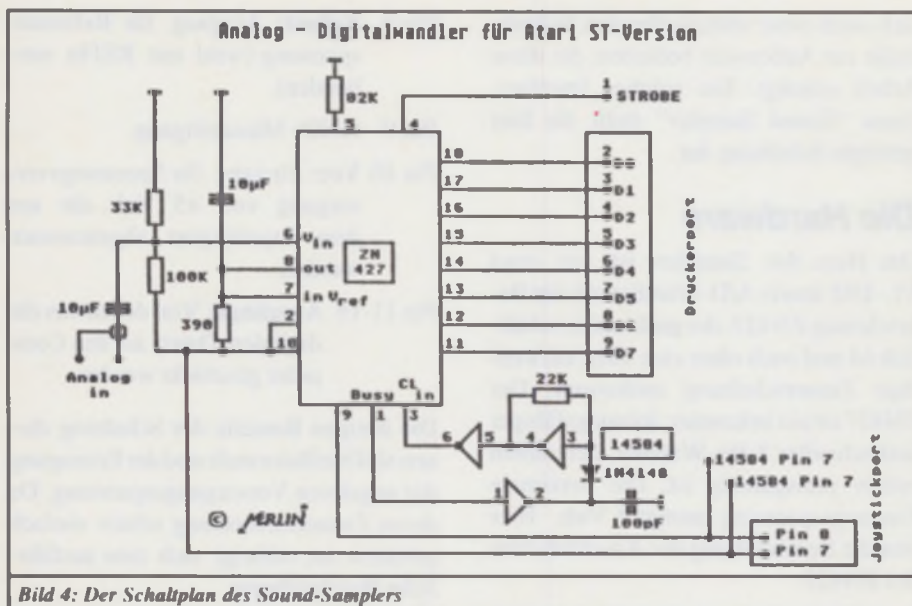
Bild 4: Der Schaltplan des Sound-Samplers
