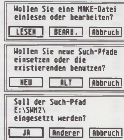
Bild 2: Bearbeiten einer MAKE-Datei
