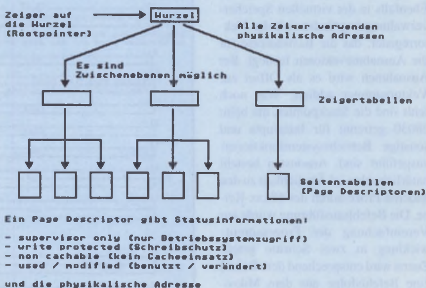
Bild 4: Die PMMU des 68030
