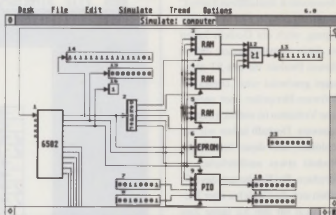
6502-Simulation mit PRODESIGN von Lissen&Beese
