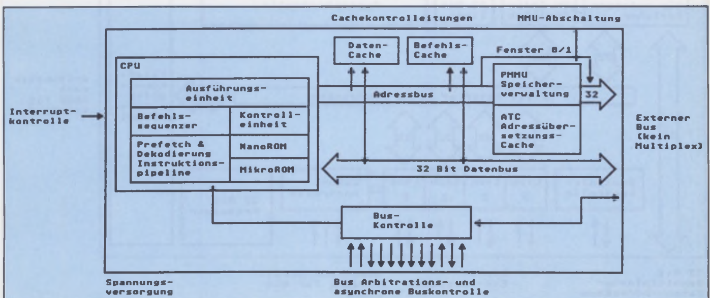
Bild 1: Die 68030 Prozessorarchitektur
