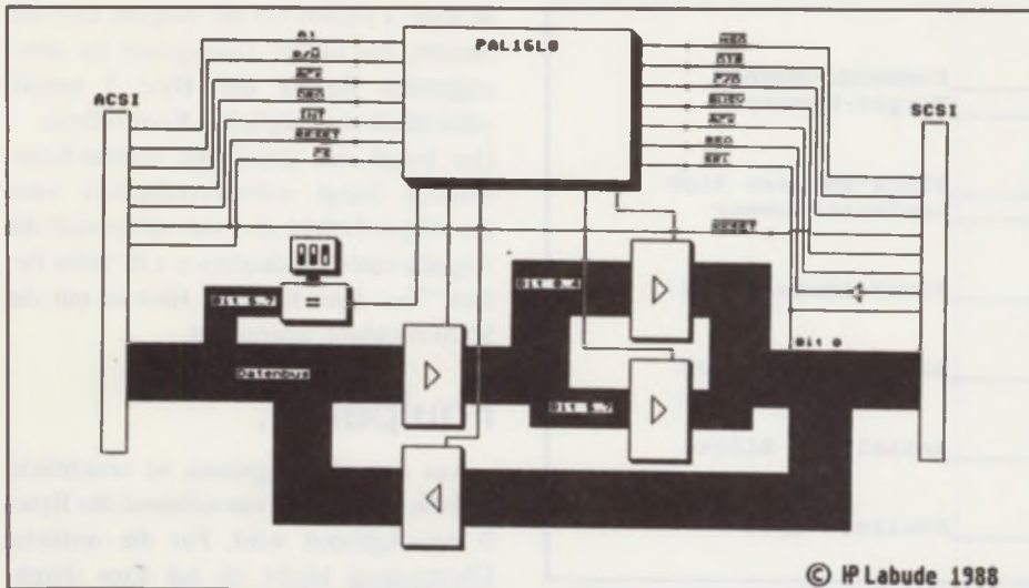
Bild 2: Blockschaltbild des ATARI-Adapters
