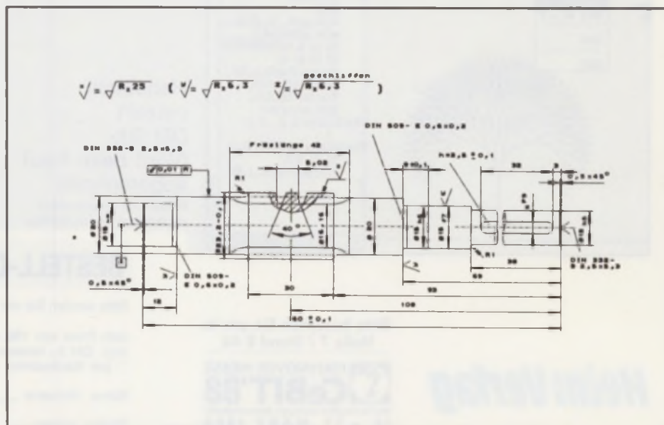
Bild 5: Ein Anwendungsbeispiel aus dem Maschinenbau
