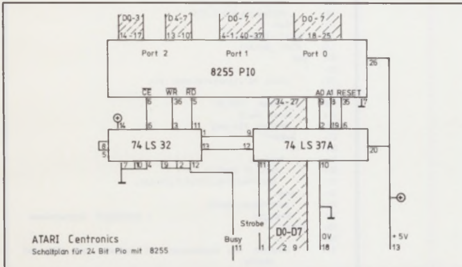
Schaltplan
