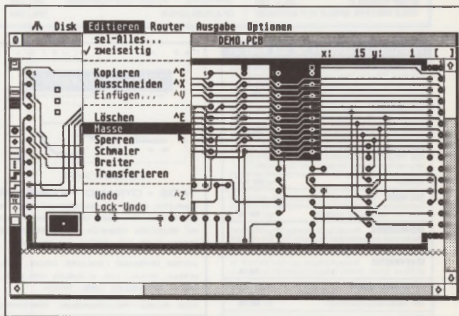
PCB - Layout mit Platinenanschnitt von 95mm x 50mm
