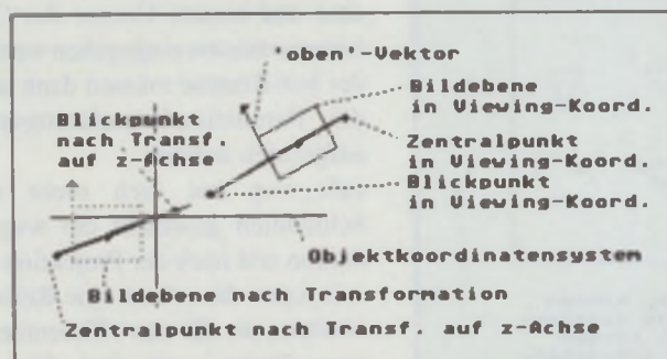
Bild 12: Viewing-Transformation In der Abbildung sind Bildebene und der Vektor zwischen Zentral und Blickpunkt, der durch den Mittelpunkt der Bildebene geht, sowohl in Viewing- wie in Objektkoordinaten gezeigt. Vor Clipping und Projektion muß die Viewing-Transformation stattfinden, wenn die Sichtachse nicht auf der z-Achse liegt. Der 'Oben'-Vektor wird nicht unbedingt benötigt.
