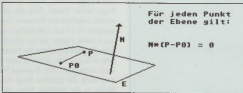
Bild 5: Ebenengleichung
