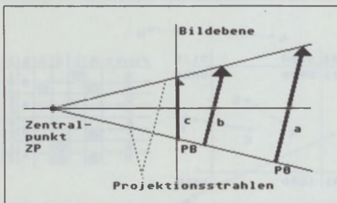
Bild 7: Zentralprojektion
