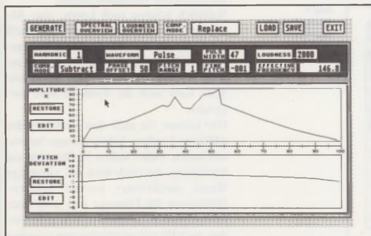
Bild 3: Additive Syn- these im S-900 Editor
