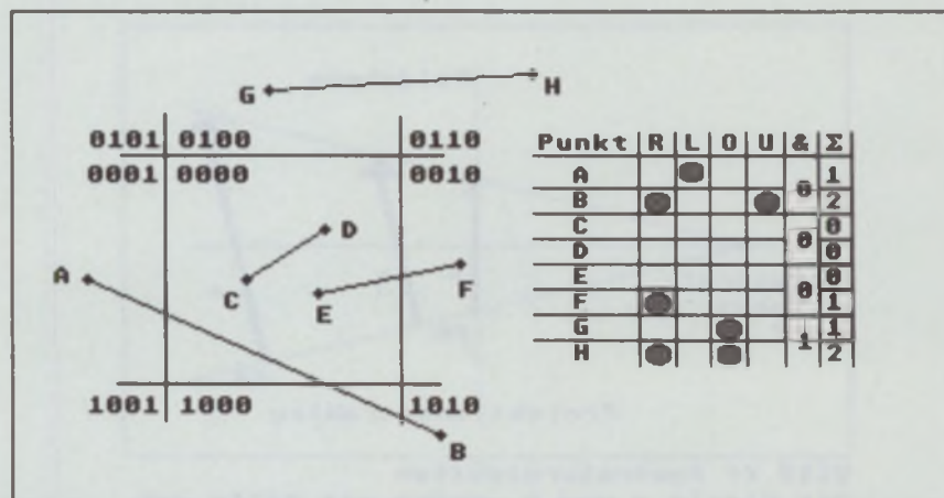
Bild 9: Endpunkt-Codes für Cohen-Sutherland-Clipping
