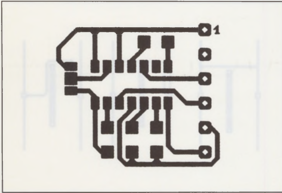
Platine für SMD - Baustein
