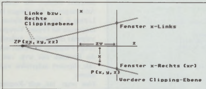
Bild 10: Vergleich von Punkten mit einer Ebene Für den x-Wert eines Punktes P auf der Clipping-Ebene gilt: x = \frac{z-zz}{zv-zz} * xr . Ein Punkt liegt also auf der Clipping-Ebene wenn x - \frac{z-zz}{zv-zz} * xr = 0 . Demnach liegt ein Punkt links von der Clippingebene, wenn der Ausdruck kleiner, rechts von der Ebene, wenn er größer null ist. Um den Rechenaufwand für die einzelnen Vergleiche zu verringern, kann man die Gleichung umformen in: x-zz*a1-a2=0 . Dabei ist a1=xr/zv-zz und a2=-a1*zz . Diese beiden Parameter haben den Vorteil, daß sie nicht von dem zu testenden Punkt abhängen und somit vorher berechnet werden können. Der eigentliche Vergleich wird damit beschleunigt. Die Parameter werden bei jeder Änderung des Fensters mit Hilfe der calc_cprm-Routine neu berechnet.
