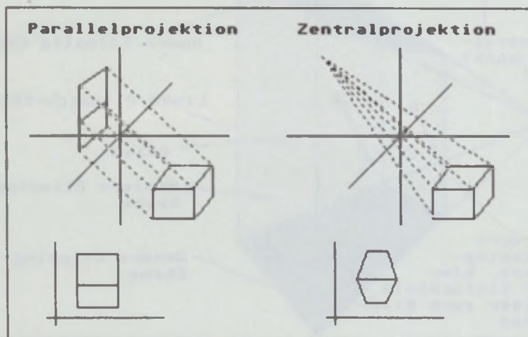
Bild 6: Projektionsarten
