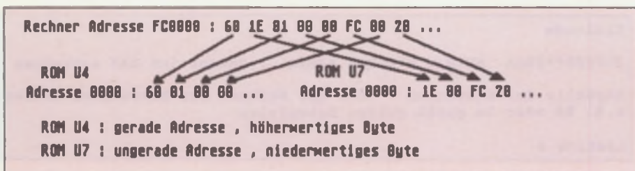
Abb. 2: Aufteilung der 16-Bit-Adressen auf die 8-Bit-ROM's
