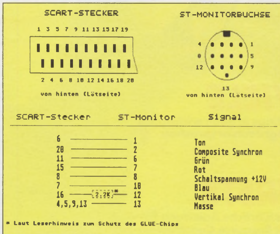
Bild 2: Anschlußbelegung eines SCART-Kabels
